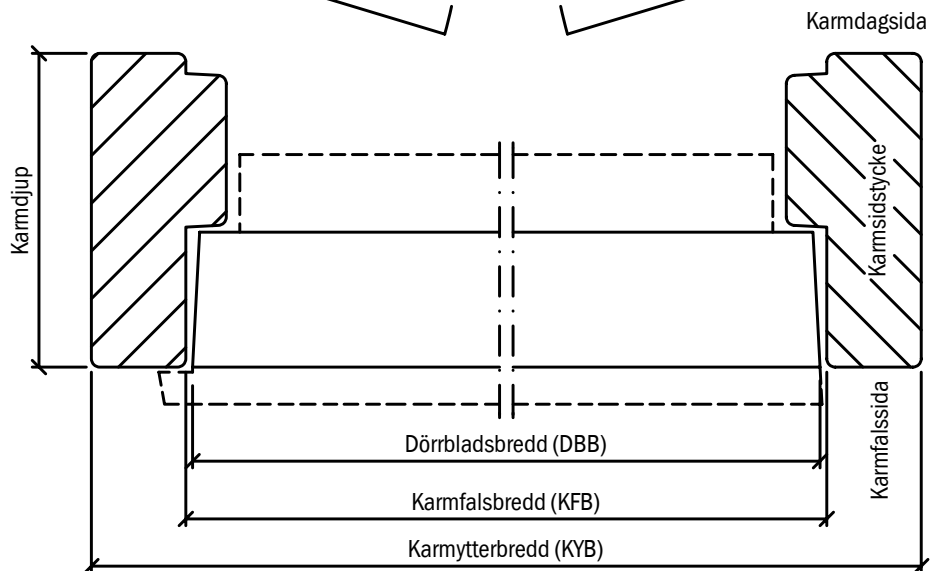
Utåtgående dörr
